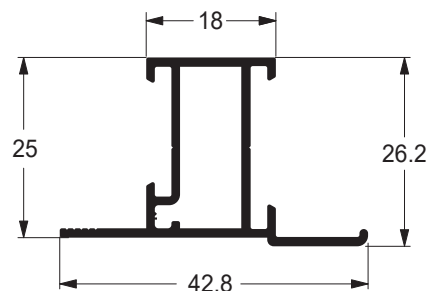
MONTANTE FOLHA SEM ESCOVA MAXIAR
