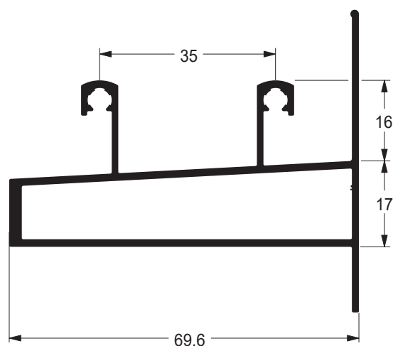
TRILHO INFERIOR C/ FIXO
