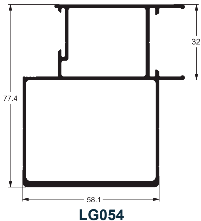
MARCO ABA LISA
