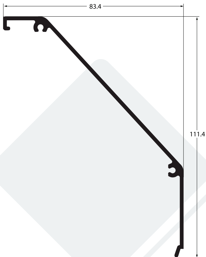
TAMPA INTERNA SUPERIOR 210MM
