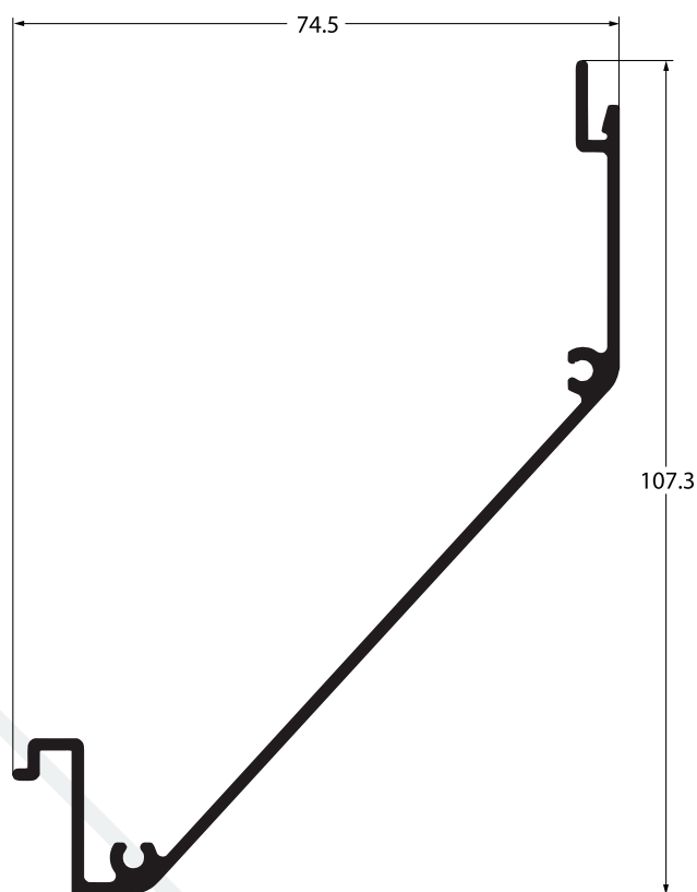
TAMPA INTERNA INFERIOR 210MM
