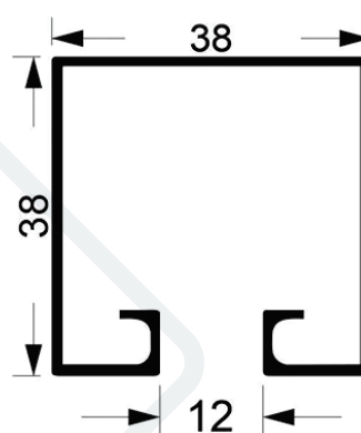
TRILHO STANLEY SUPERIOR 38MM
