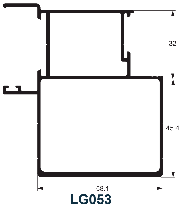
MARCO ABA LISA
