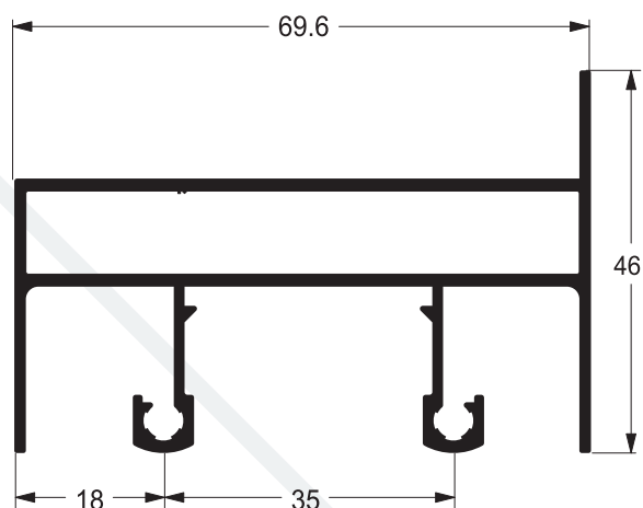
TRAVESSA BANDEIRA/ MARCO/CORRER 2
