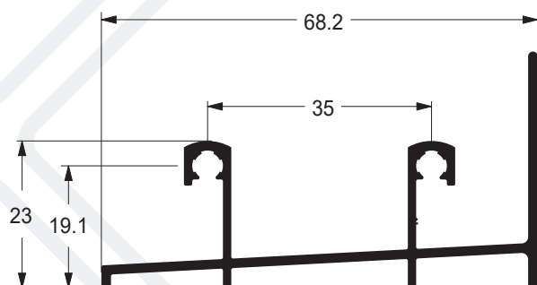
TRILHO INFERIOR PORTA 2 FOLHAS
