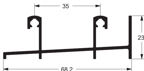
MARCO INFERIOR 2 FOLHAS
