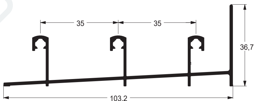
MARCO INFERIOR PORTA 3 FOLHAS
