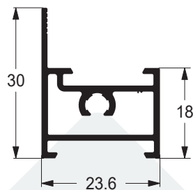
MONTANTE FOLHA COM OLHAL MAXIAR
